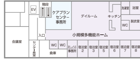
2階平面図
